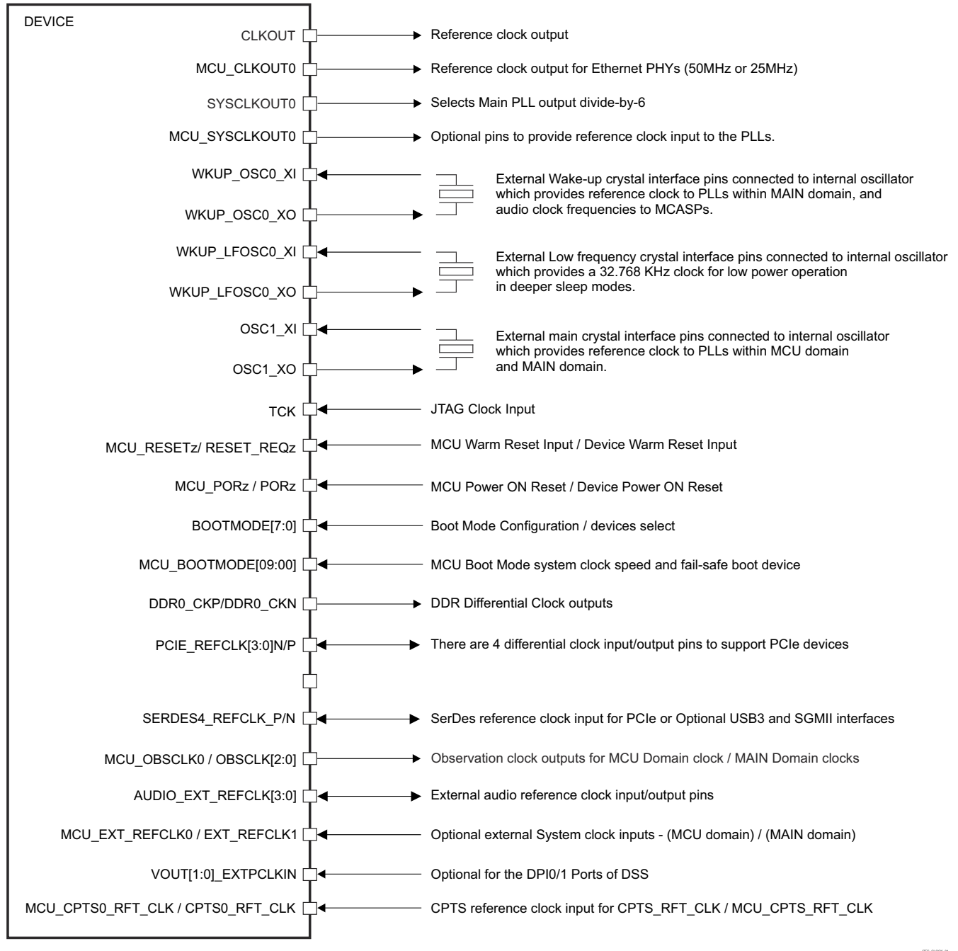
图 7-22. Input Clocks Interface
