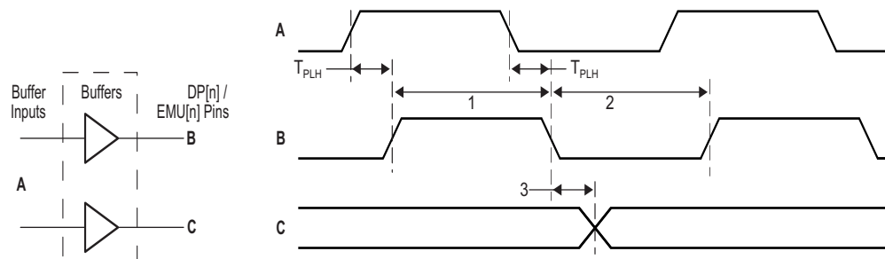
图 5-68. Trace Timing
