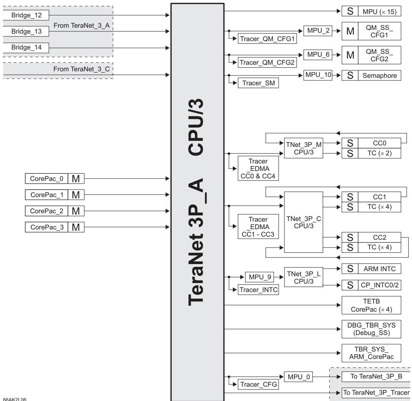
图 6-74. TeraNet 3P_A
