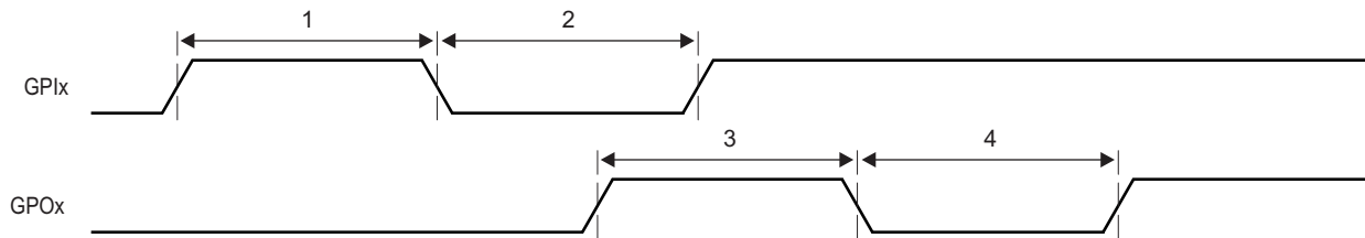
图 5-58. GPIO Timing
