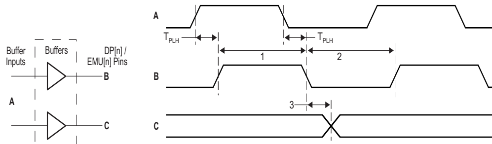
图 11-57. Trace Timing
