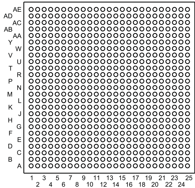
图 4-1. ABY FCBGA-N625 Package (Bottom View)
