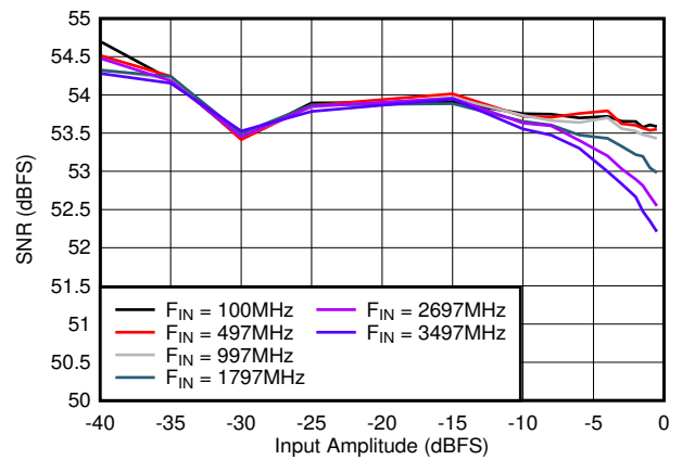
图 7-30. SNR vs Input Amplitude
