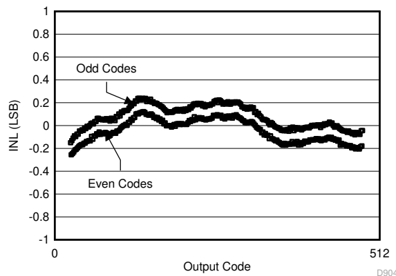
图 7-2. INL vs Code
