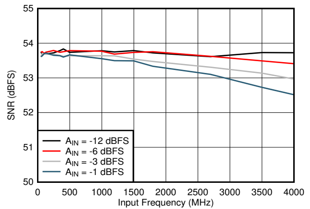
图 7-16. SNR vs Input Frequency
