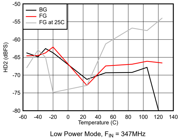
图 7-43. HD2 vs Temperature
