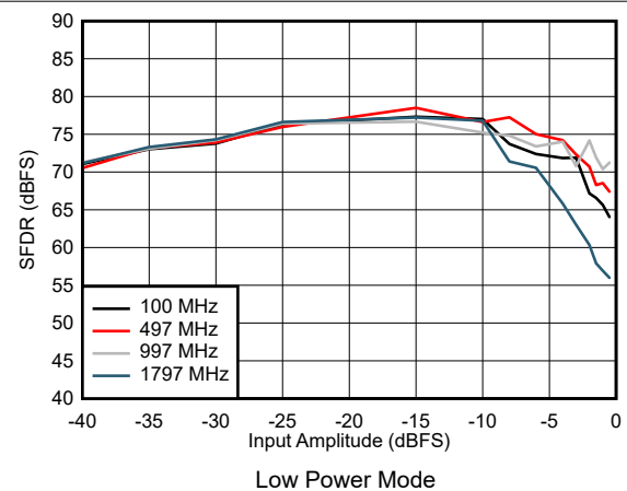
图 7-30. SFDR vs Input Amplitude
