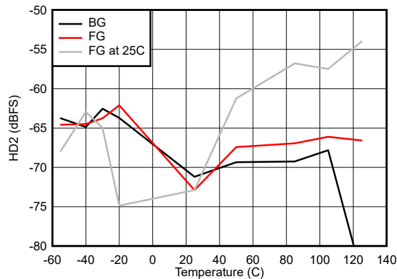
图 7-43. HD2 vs Temperature
