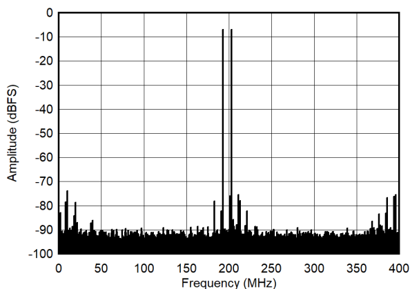
图 7-52. Dual Tone FFT at 998 MHz
