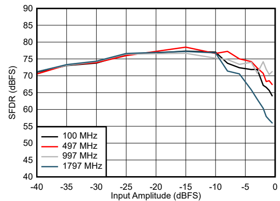
图 7-30. SFDR vs Input Amplitude
