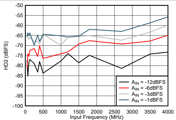
图 7-18. HD2 vs Input Frequency
