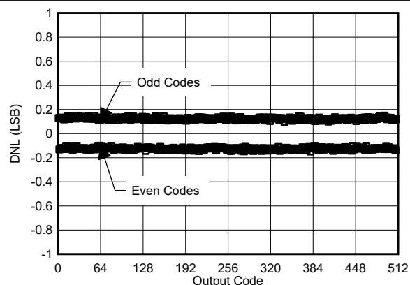
图 7-1. DNL vs Code
