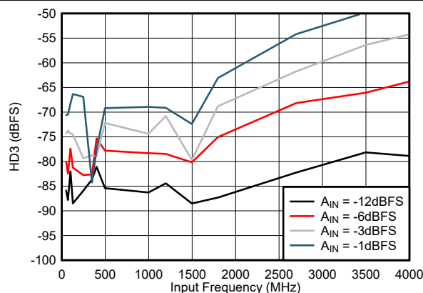
图 7-19. HD3 vs Input Frequency
