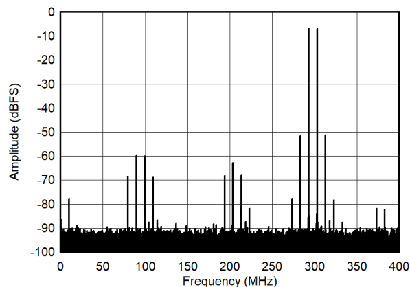
图 7-55. Dual Tone FFT at 2698 MHz
