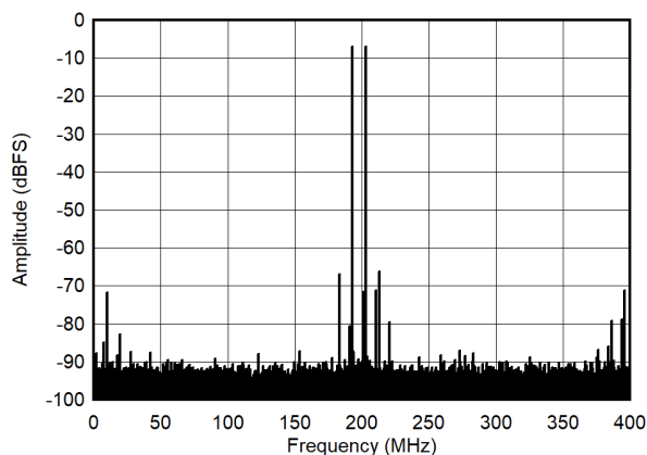
图 7-53. Dual Tone FFT at 1798 MHz
