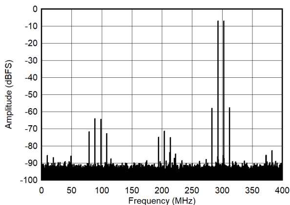
图 7-54. Dual Tone FFT at 2698 MHz
