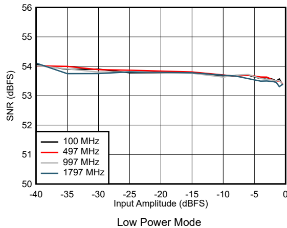
图 7-31. SNR vs Input Amplitude
