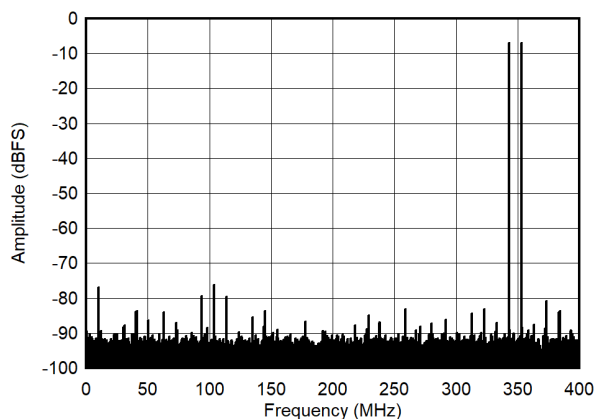
图 7-51. Dual Tone FFT at 348 MHz
