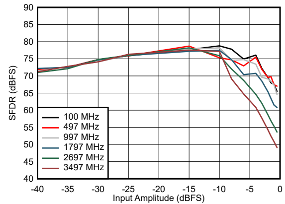
图 7-28. SFDR vs Input Amplitude
