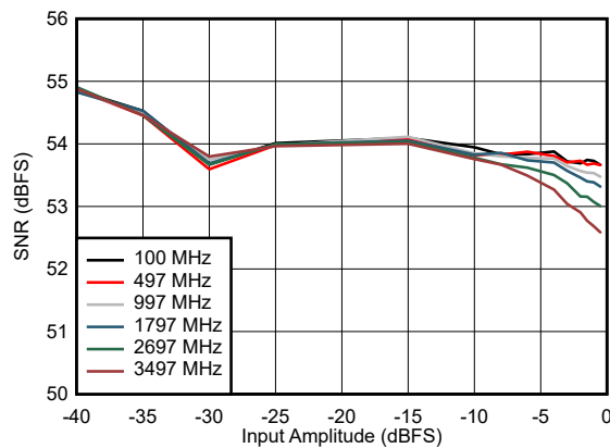
图 7-29. SNR vs Input Amplitude
