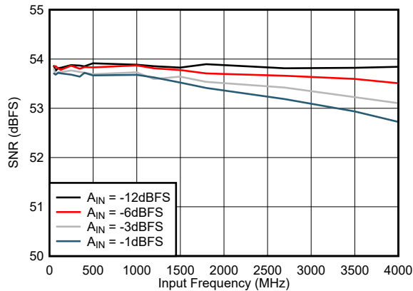
图 7-15. SNR vs Input Frequency
