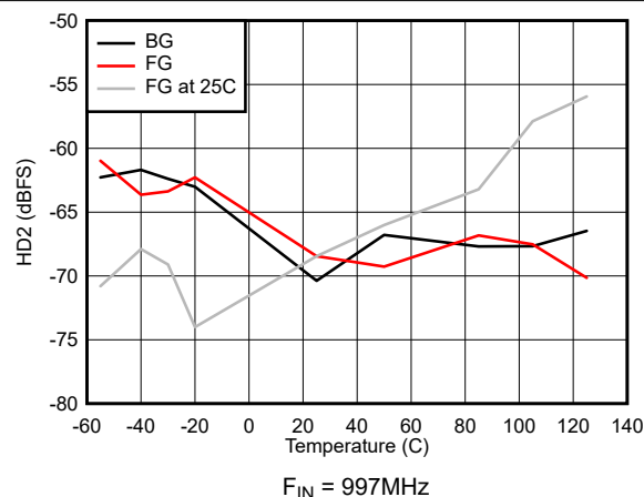
图 7-37. HD2 vs Temperature
