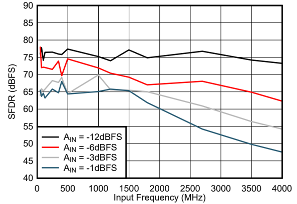
图 7-14. SFDR vs Input Frequency
