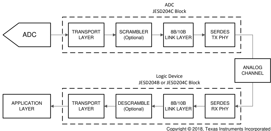
图 8-7. Simplified 8B/10B Encoded JESD204C Interface Diagram
