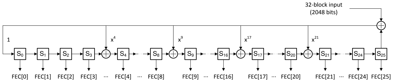
图 8-10. FEC Parity Bit Generator
