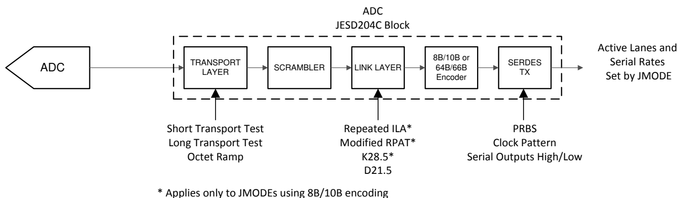
图 8-14. Test Mode Insertion Points
