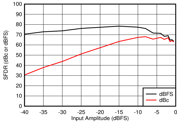
图 7-31. SFDR vs Input Amplitude
