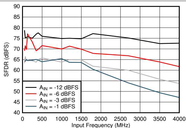
图 7-15. SFDR vs Input Frequency
