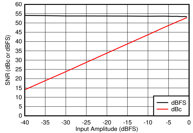
图 7-32. SNR vs Input Amplitude
