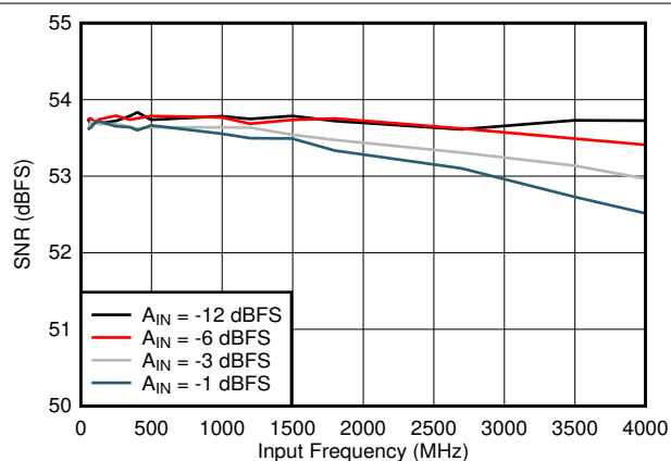
图 7-16. SNR vs Input Frequency
