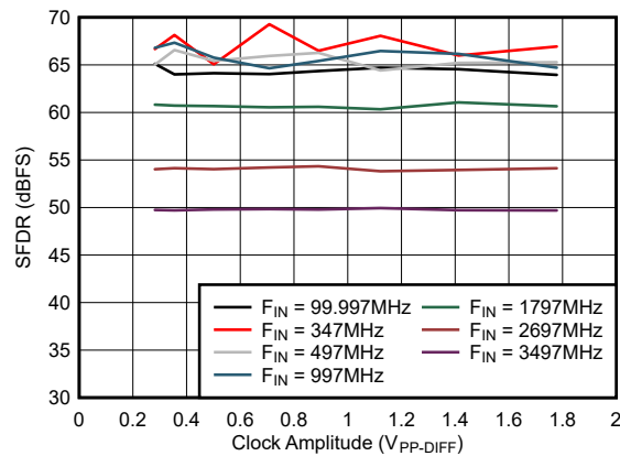
图 7-33. SFDR vs Clock Amplitude
