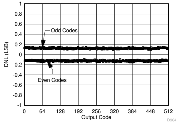
图 7-1. DNL vs Code
