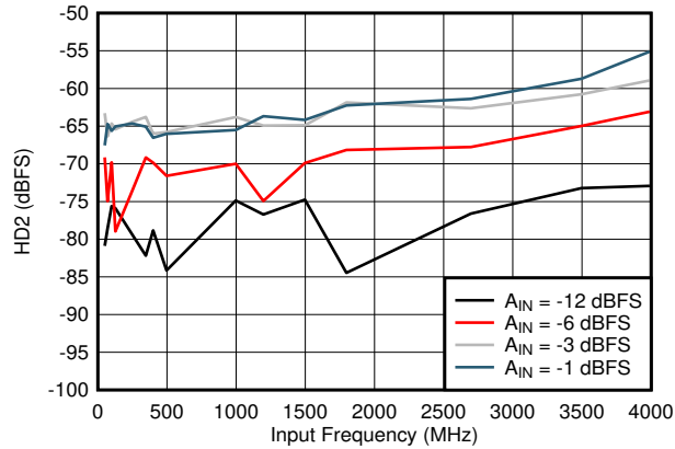
图 7-19. HD2 vs Input Frequency
