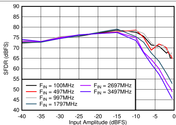
图 7-29. SFDR vs Input Amplitude
