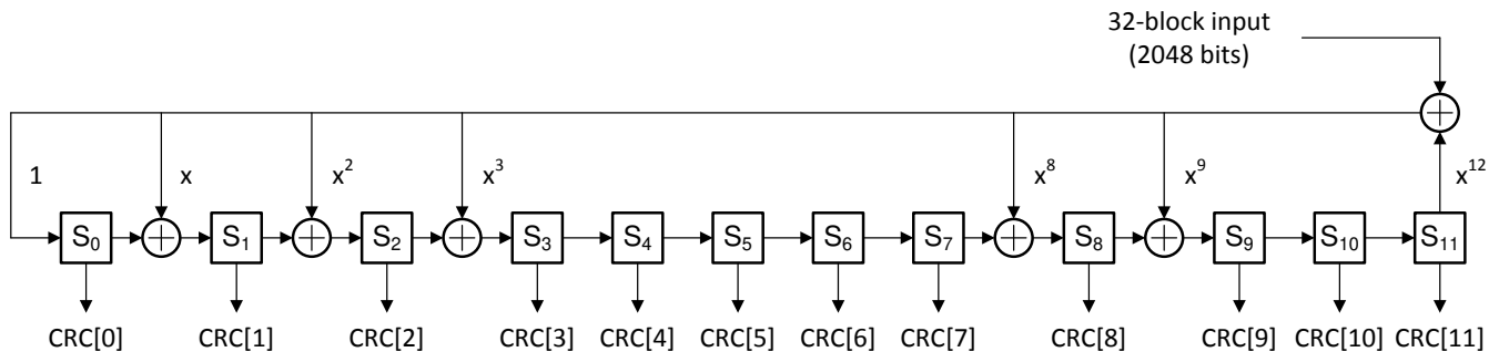
图 8-9. CRC-12 Parity Bit Generator
