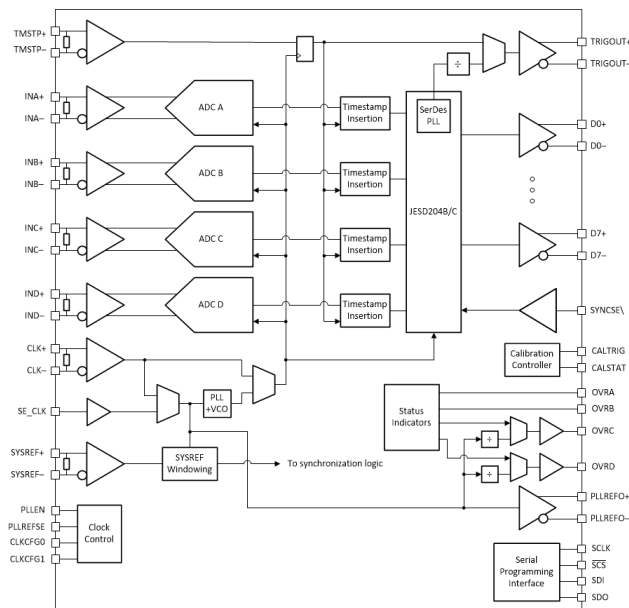
四通道器件方框图
