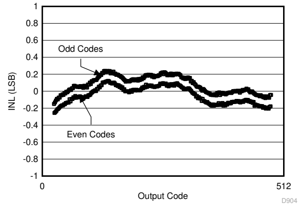
图 7-2. INL vs Code
