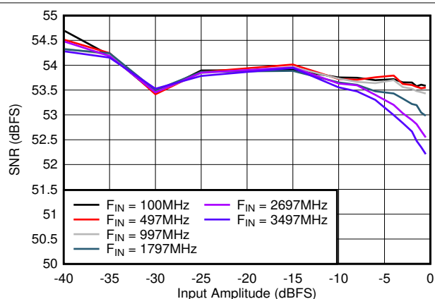
图 7-30. SNR vs Input Amplitude
