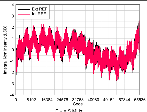
图 6-20. INL vs Code
