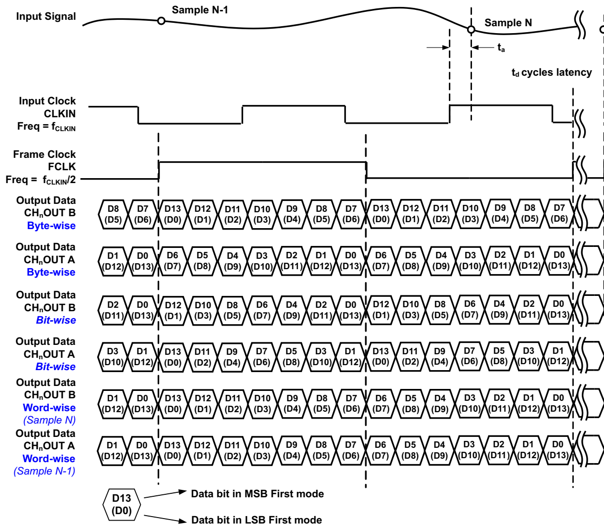
图 54. 14-Bit Word Wise
