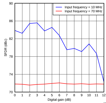
图 17. SFDR vs Digital Gain
