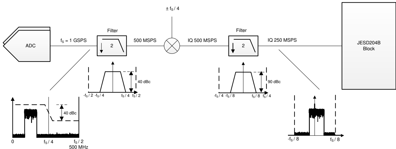
图 7-9. Operating Mode 0
