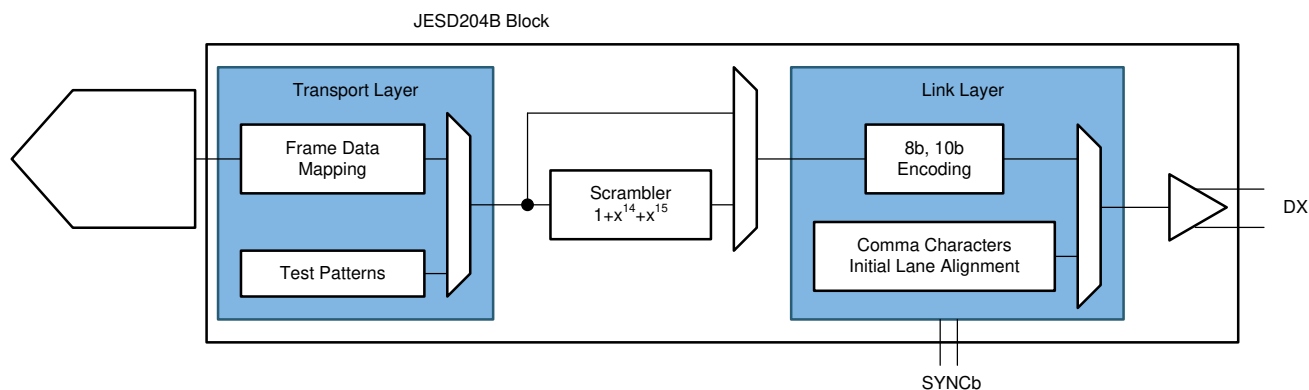
图 7-22. JESD Interface Block Diagram
