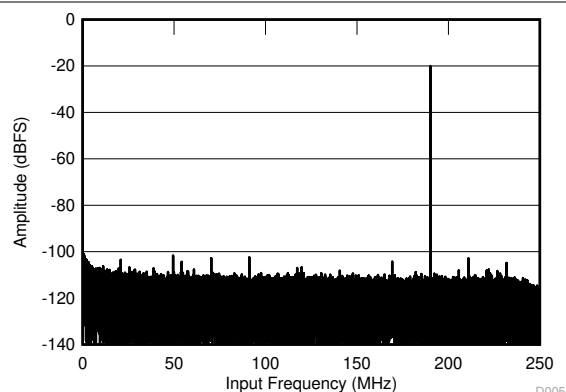
图 6-4. FFT for 190-MHz Input Signal
