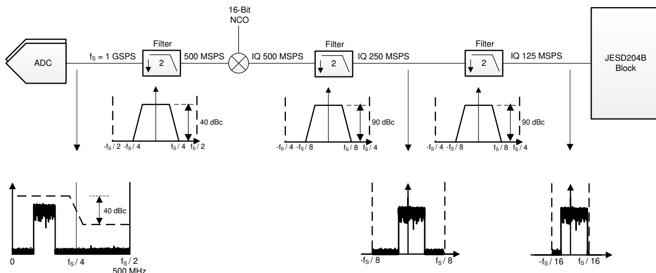
图 7-14. Operating Mode 6
