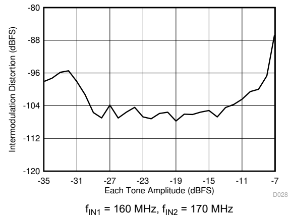
图 6-29. IMD vs Input Amplitude
