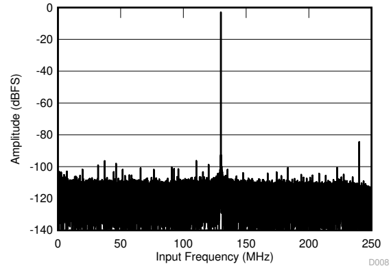
图 6-9. FFT for 370-MHz Input Signal
