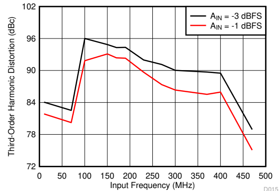
图 6-16. HD3 vs Input Frequency
