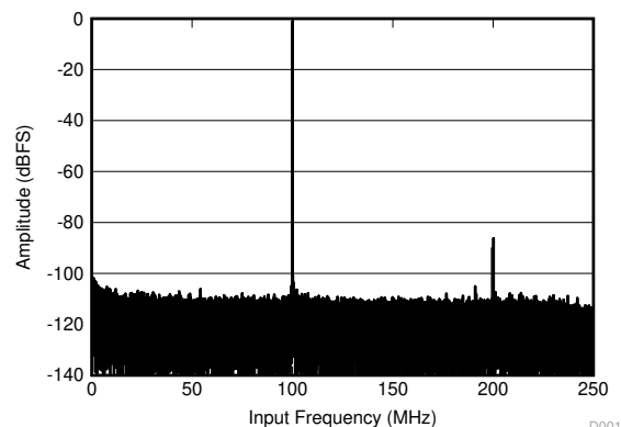
图 6-2. FFT for 100-MHz Input Signal
