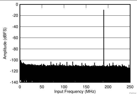
图 6-3. FFT for 190-MHz Input Signal
