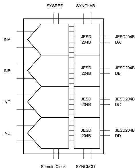
图 7-21. JESD204B Transmitter Block
