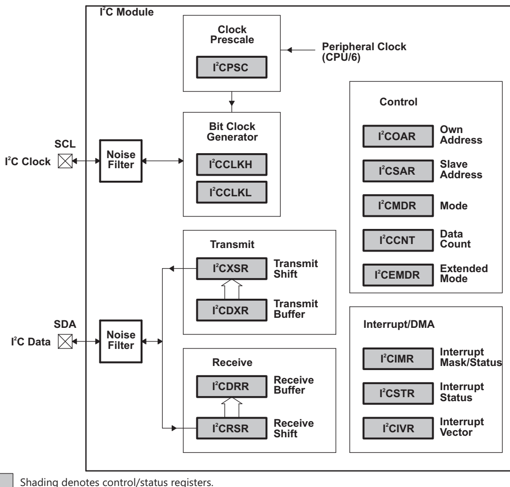
图 10-30. I²C Module Block Diagram
