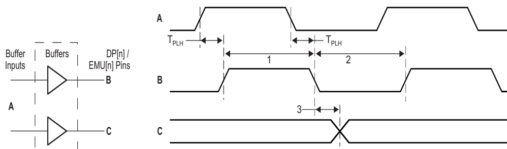
图 10-55. Trace Timing
