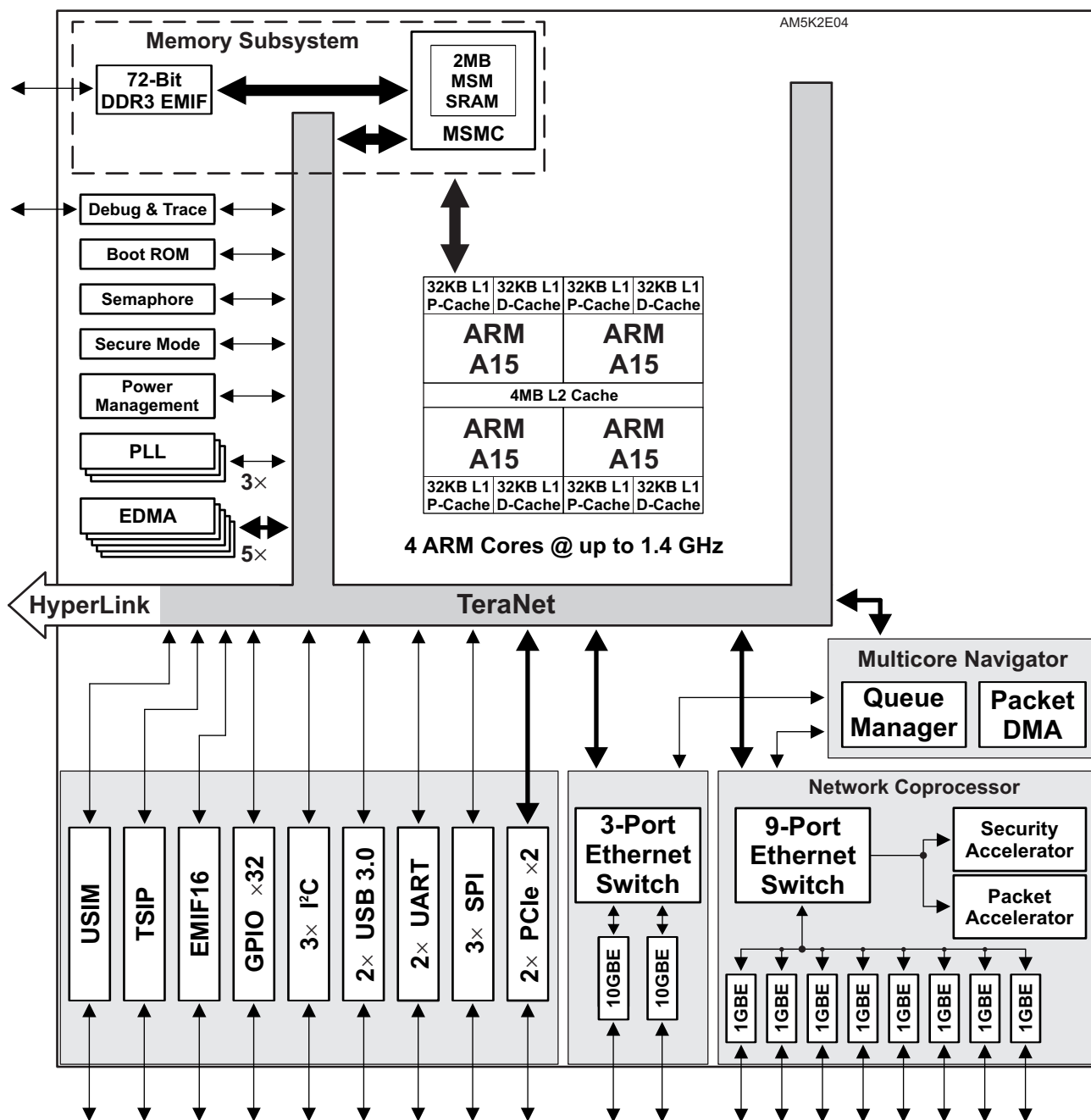
图 1-1. AM5K2E04 功能框图
