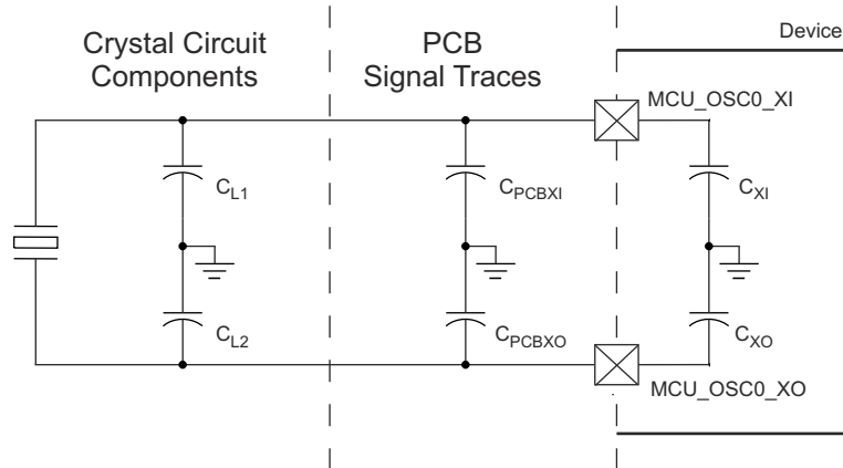
图 7-17. Load Capacitance
