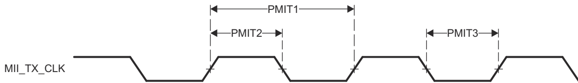
图 7-103. PRU_ICSSG MII[x]_TX_CLK Timing
