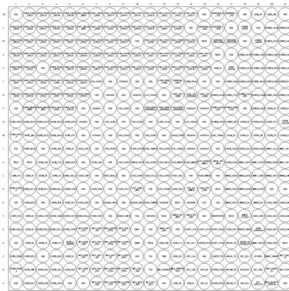
图 6-1. ALV FCBGA-N441 Pin Diagram (Bottom View)
