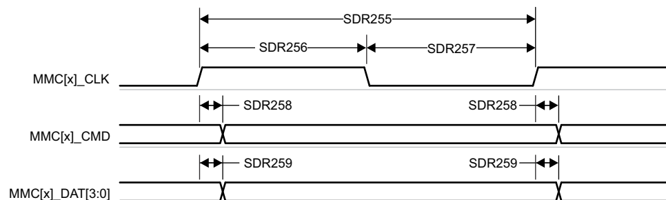
图 7-71. MMC1 - UHS-I SDR25 - Transmit Mode
