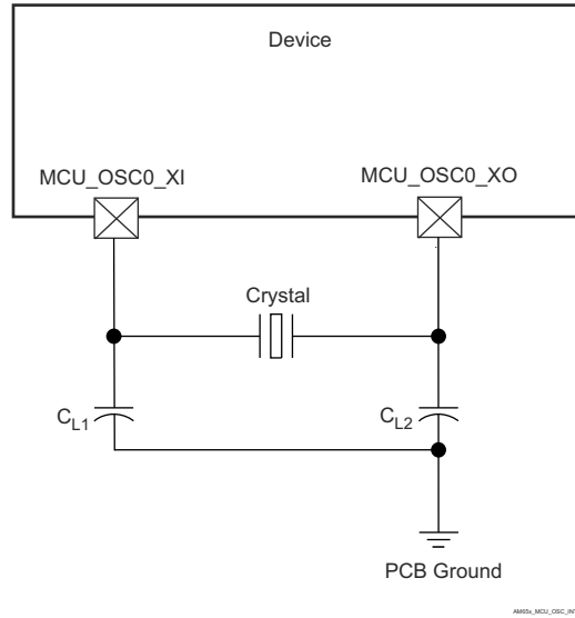
图 7-15. MCU_OSC0 Crystal Implementation
