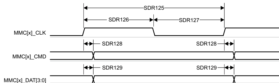
图 7-69. MMC1 - UHS-I SDR12 - Transmit Mode
