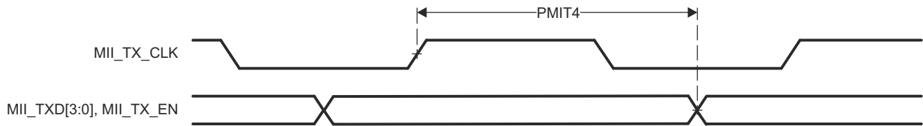
图 7-104. PRU_ICSSG MII[x]_TXD[3:0], MII[x]_TX_EN Timing
