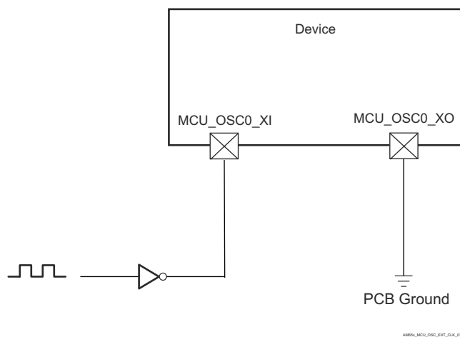
图 7-19. 1.8-V LVCMOS-Compatible Clock Input
