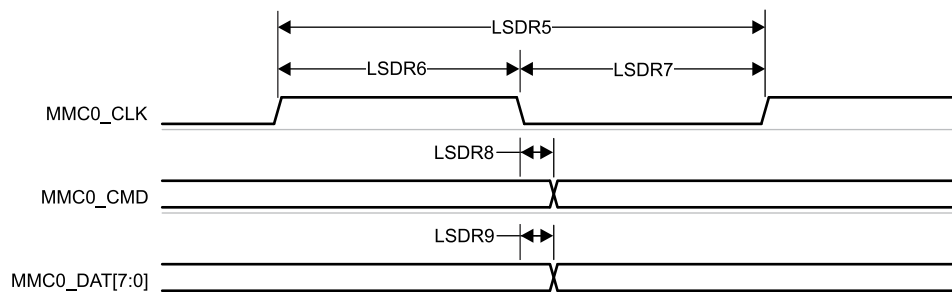
图 7-58. MMC0 – Legacy SDR – Transmit Mode
