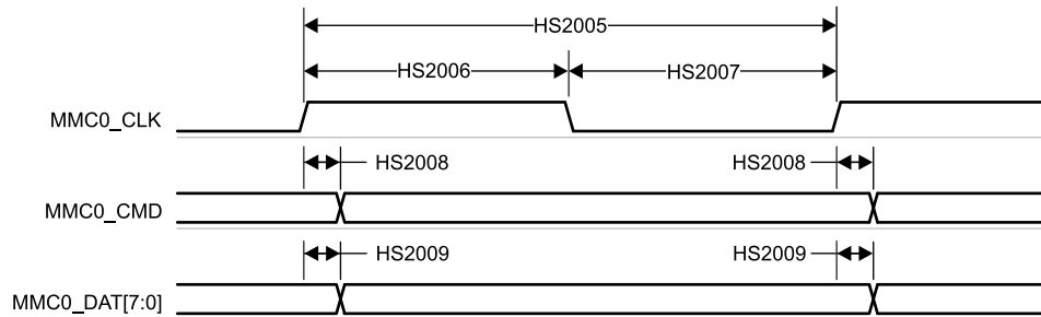
图 7-63. MMC0 - HS200 Mode - Transmit Mode
