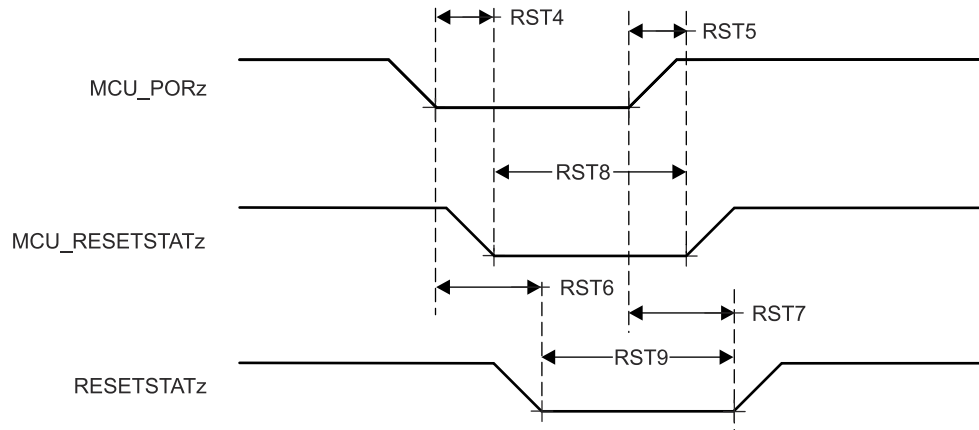
图 7-6. MCU_RESETSTATz, and RESETSTATz Switching Characteristics
