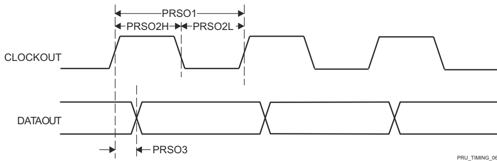
图 7-88. PRU_ICSSG PRU Shift Out Timing
