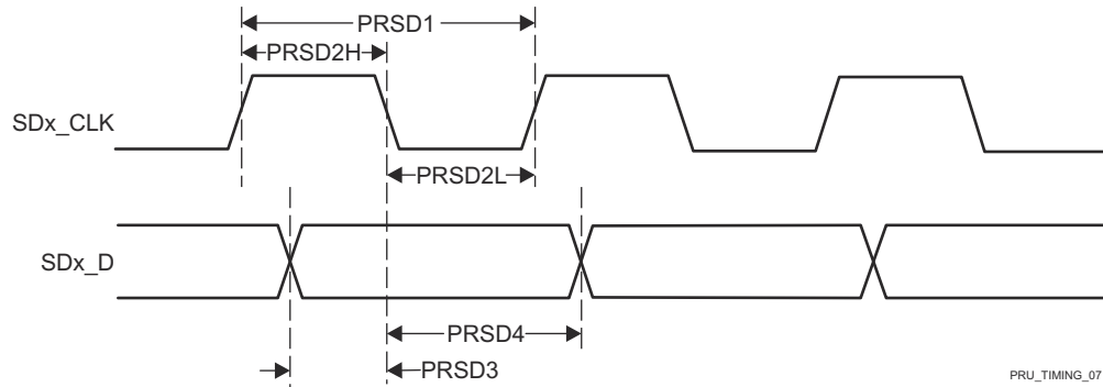
图 7-89. PRU_ICSSG PRU SD_CLK Falling Active Edge
