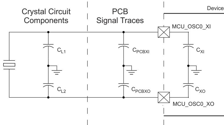
图 7-17. Load Capacitance
