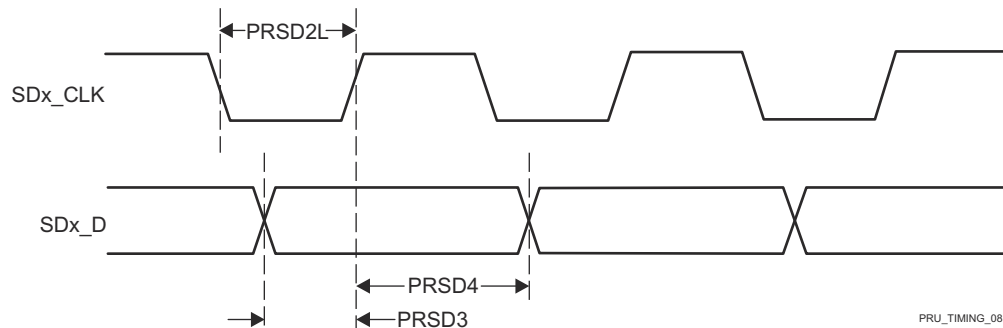
图 7-90. PRU_ICSSG PRU SD_CLK Rising Active Edge
