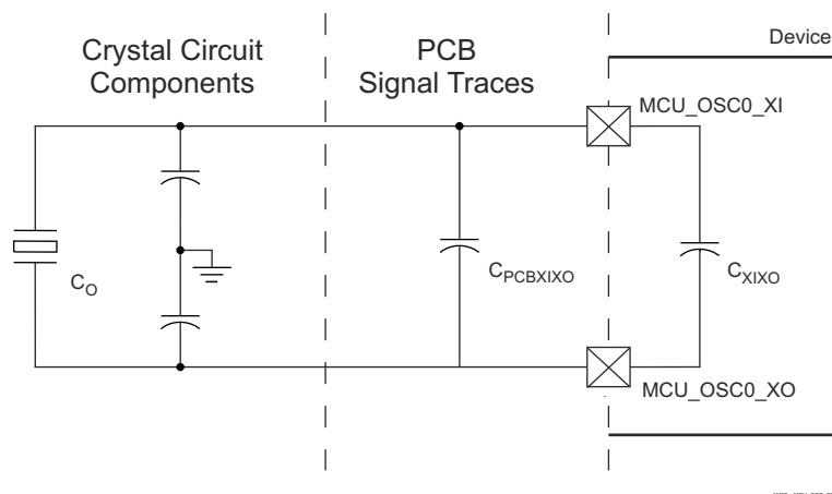
图 7-18. Shunt Capacitance
