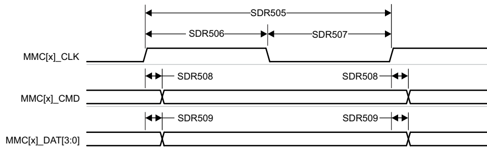
图 7-72. MMC1 - UHS-I SDR50 - Transmit Mode
