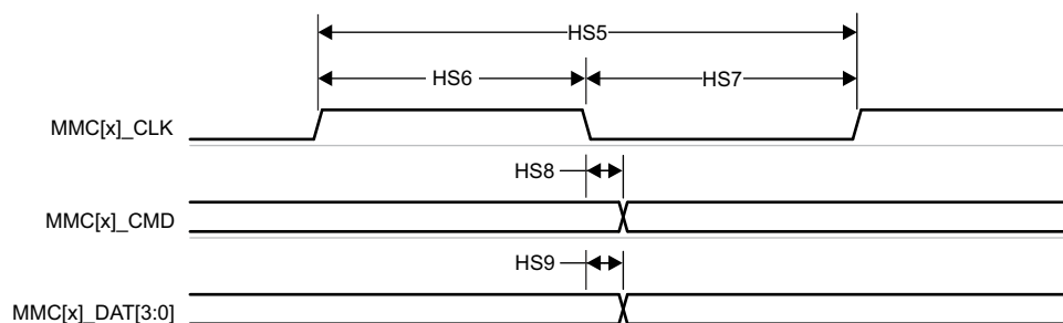
图 7-67. MMC1 - High Speed - Transmit Mode
