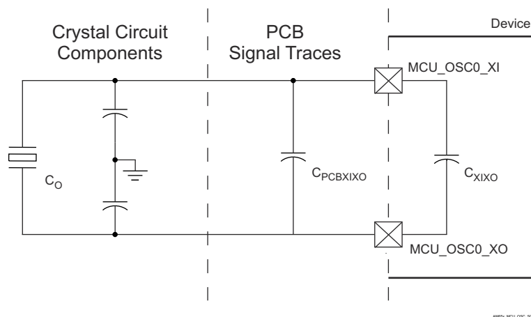
图 7-18. Shunt Capacitance
