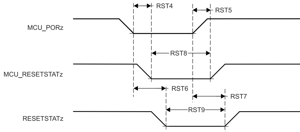
图 7-6. MCU_RESETSTATz, and RESETSTATz Switching Characteristics
