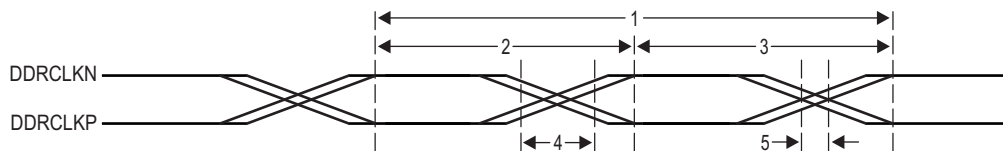
图 10-25. DDR3 PLL DDRCLK Timing
