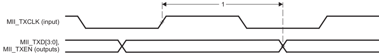
图 7-108. PRU-ICSS MII_TXD[3:0], MII_TXEN Timing
