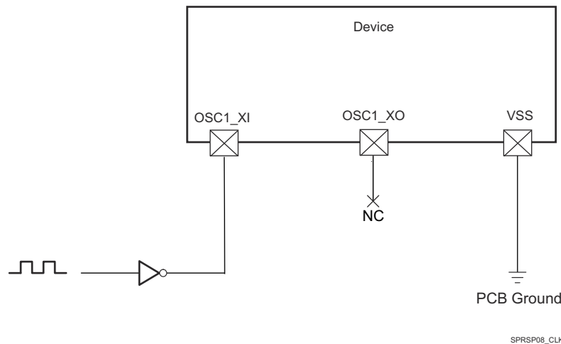
图 7-22. 1.8-V LVCMOS-Compatible Clock Input
