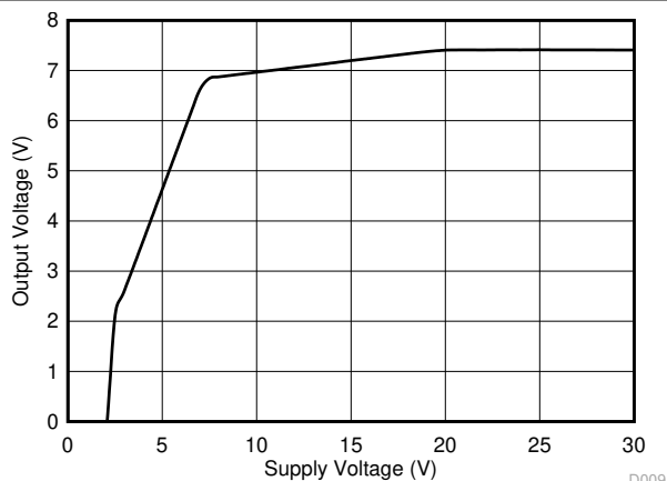
图 7-8. V_{OUT} vs V_{DD}
