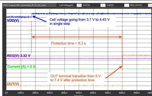
图 9-4. Overvoltage Protection
