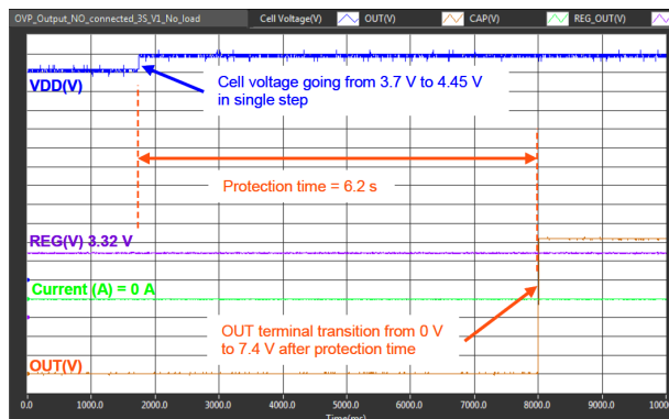
图 9-4. Overvoltage Protection
