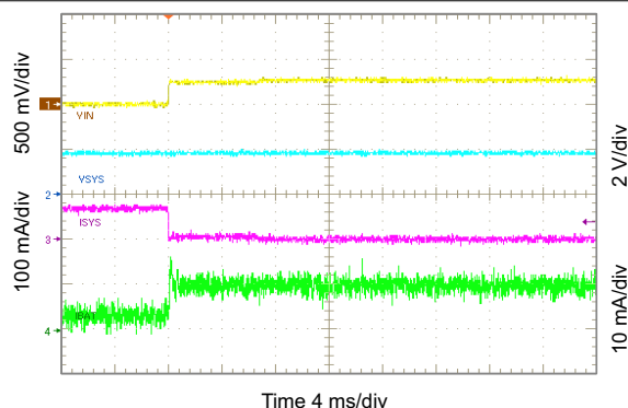
图 10-5. Exiting DPPM Mode
