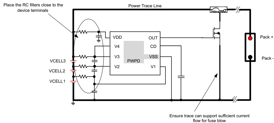
图 11-1. Layout Example
