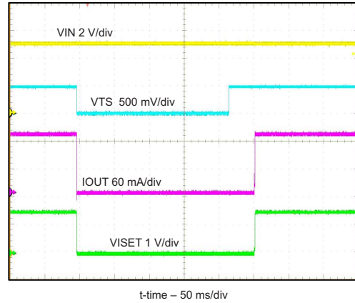
图 6. TS Enable and Disable
