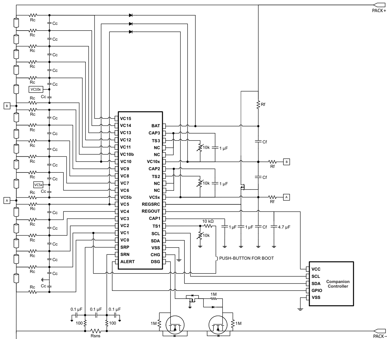
图 9-3. BQ76940 与 BQ78350 伴生控制器 IC
