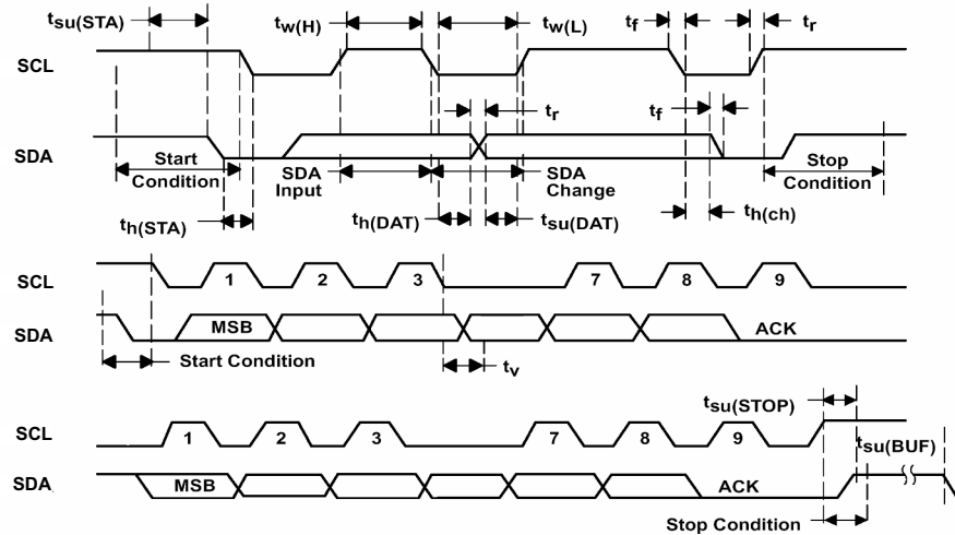
图 7-1. I²C Timing
