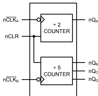
图 7-2. Functional Pinout
