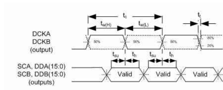
图 6-9. DMD LVDS Interface
