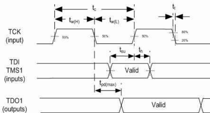
图 6-4. I/O Boundary Scan
