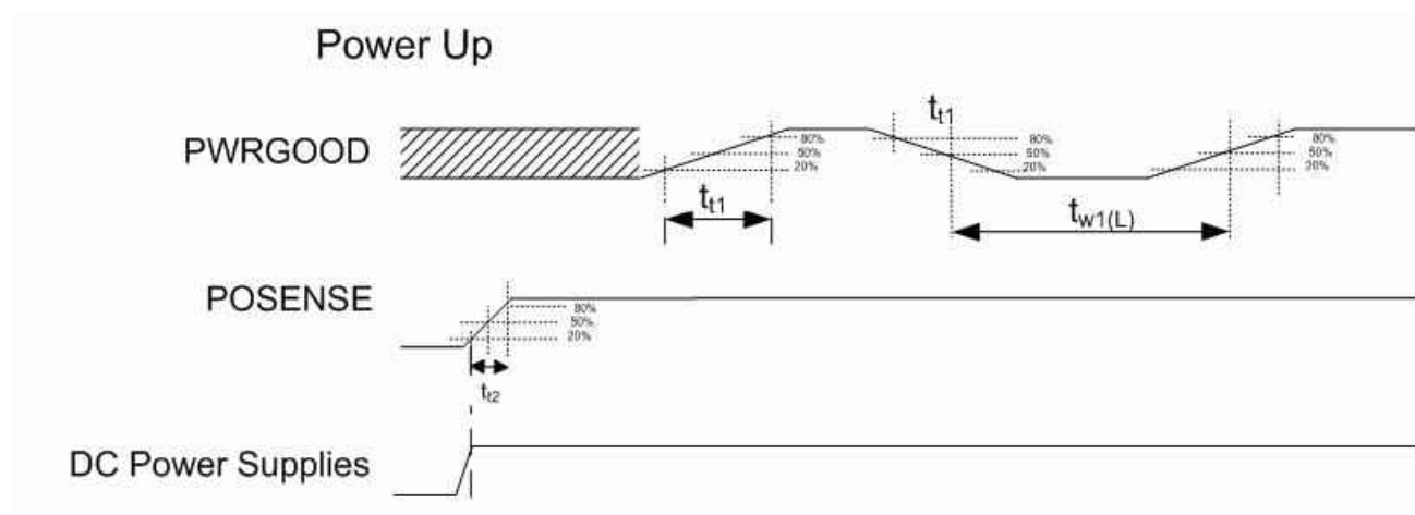
图 6-2. Power Up
