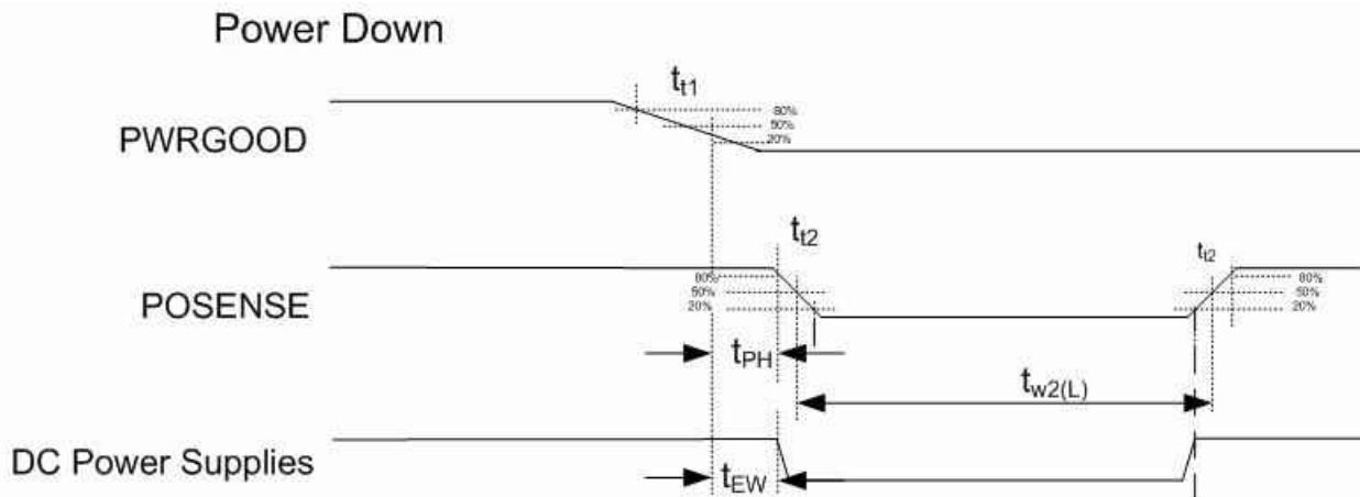
图 6-3. Power Down
