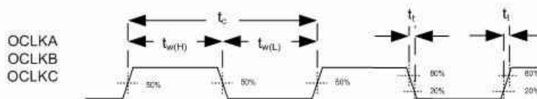
图 6-5. Programmable Output Clocks
