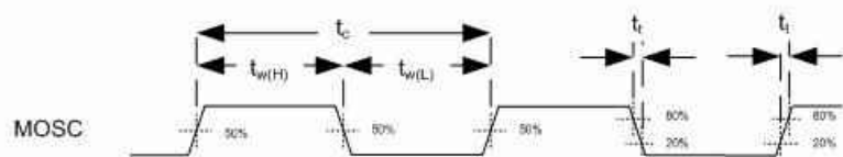
图 6-1. System Oscillators
