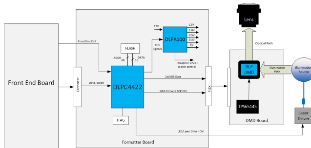
图 1. 典型应用图
