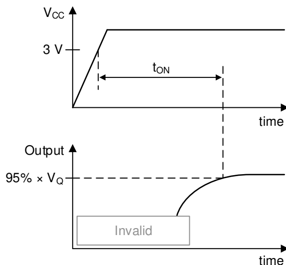
图 7-4. t_{ON} Definition
