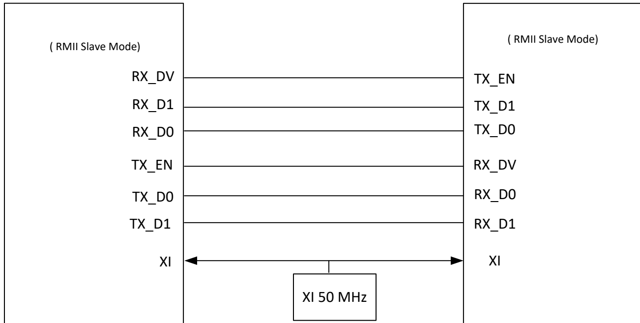
图 7-1. RMII Repeater Mode
