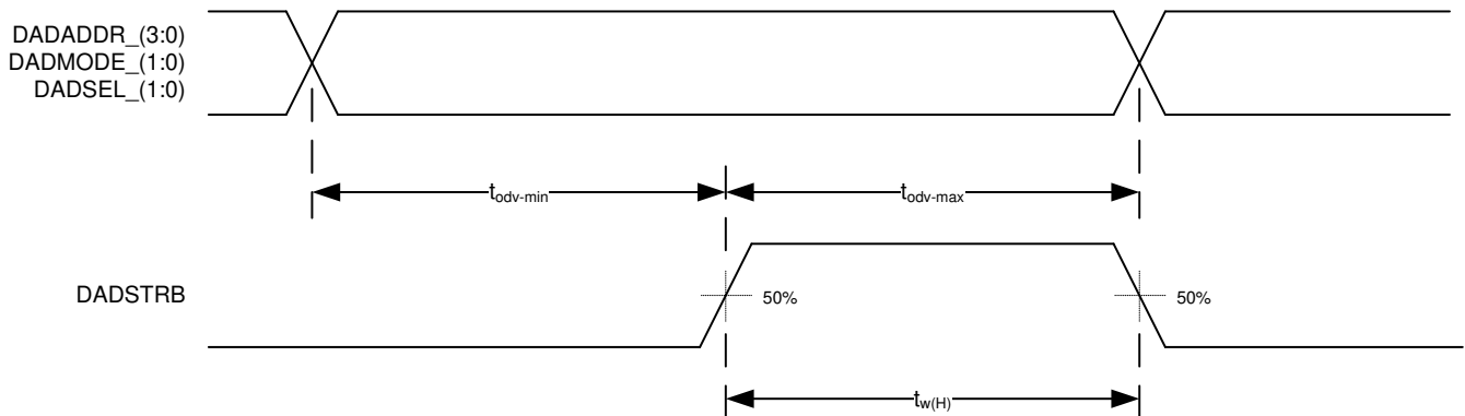
图 6-12. DMD Interface Timing
