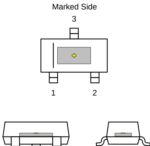
图 18. SOT-23 (DBZ) 封装
