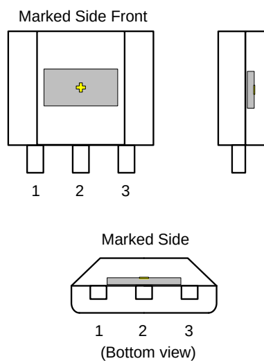
图 19. SIP (LPG) 封装
