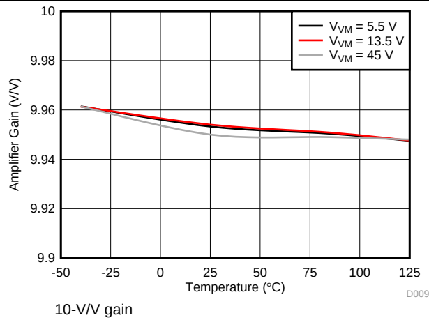
图 11. Amplifier Gain
