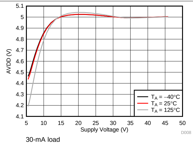
图 10. AVDD Regulator
