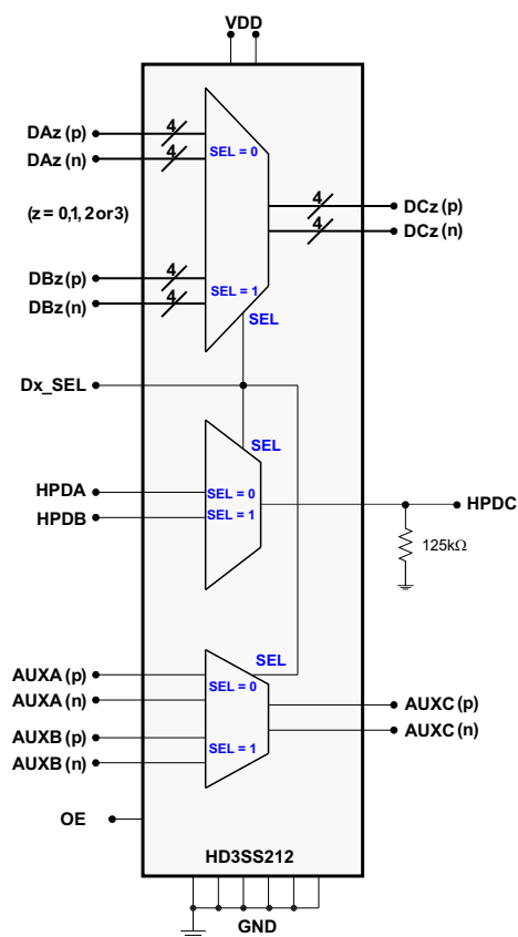
功能方框图
