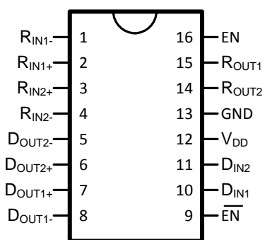
双列直插式
