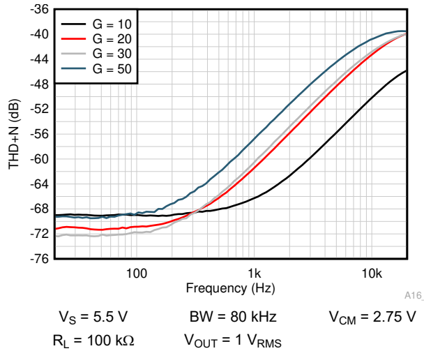
图 7-37. THD + N Frequency
