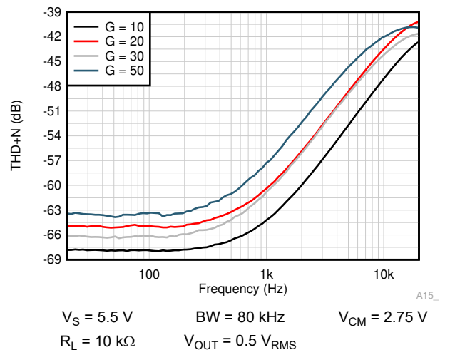
图 7-36. THD + N Frequency
