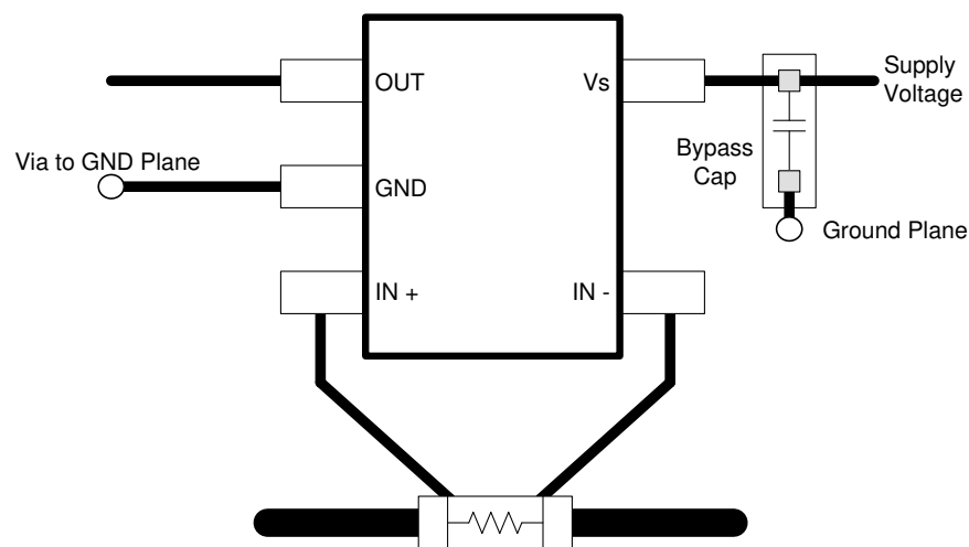
图 10-1. INA293A-Q1 Recommended Layout
