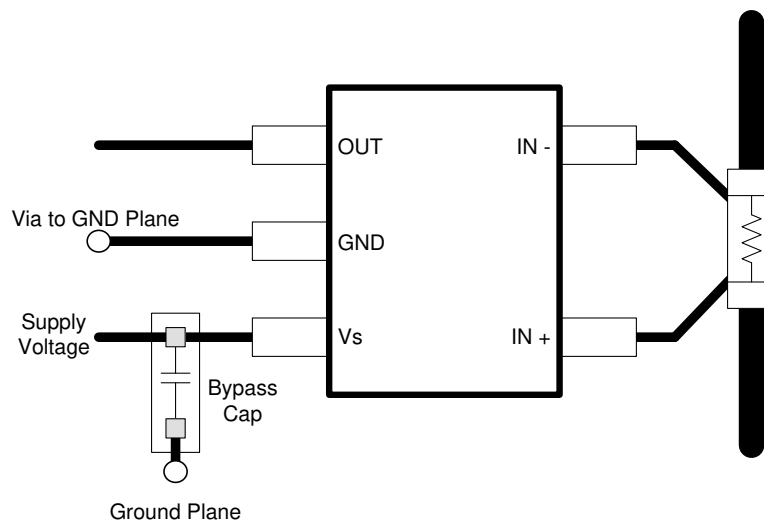
图 10-2. INA293B-Q1 Recommended Layout
