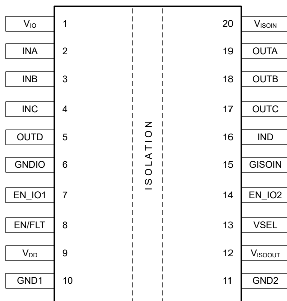
图 6-1. ISOW7741 DFM Package 20-Pin SOIC-WB Top View
