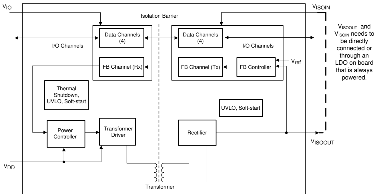
图 9-1. Block Diagram
