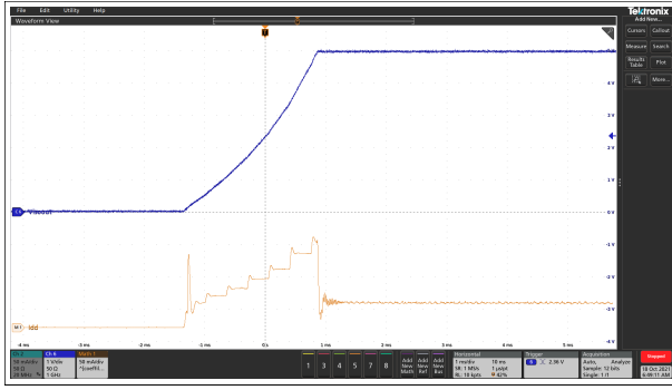
V_{DD} = 5\text{ V} V_{ISOOUT} = 5\text{ V} 10 uF Capacitor on V_{ISOOUT}
