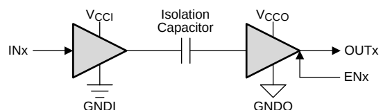
简化原理图
