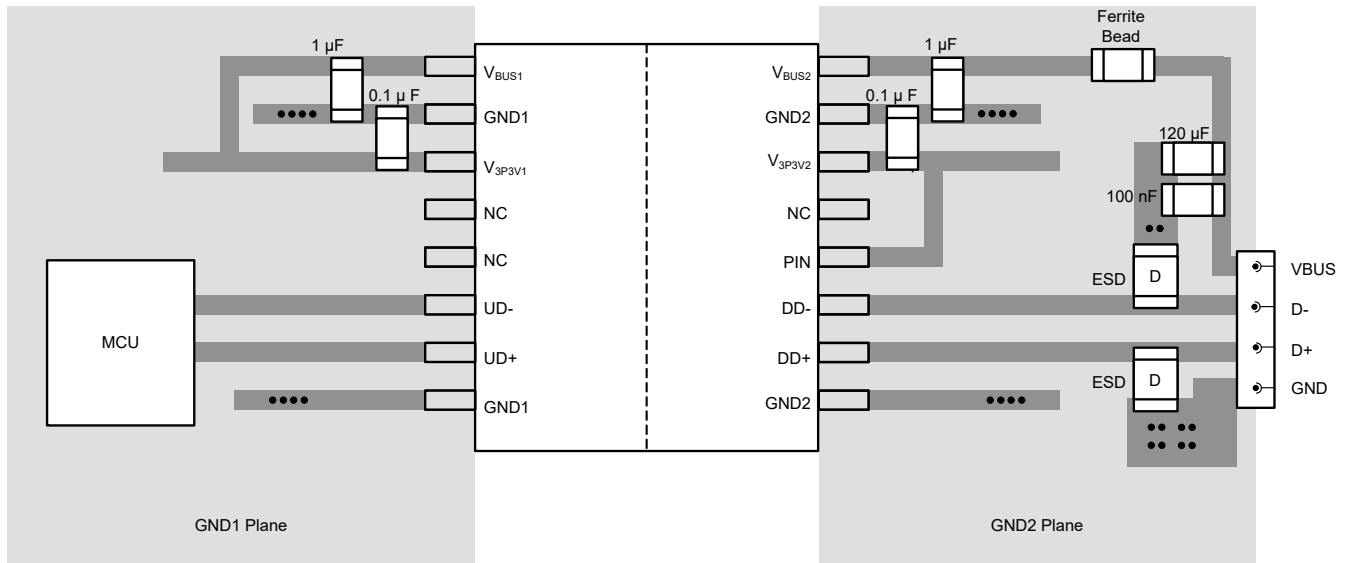
图 11-1. Layout Example for ISOUSB111
