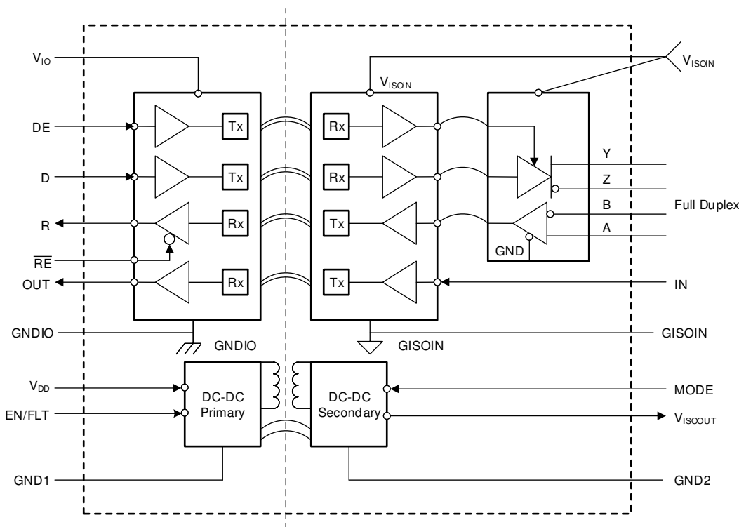
图 10-1. Block Diagram
