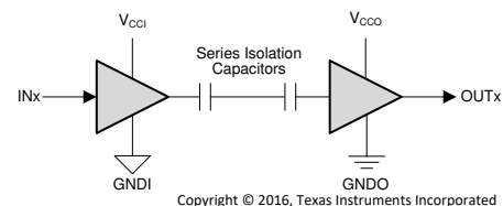
简化原理图
