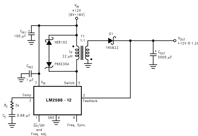
反激式稳压器
