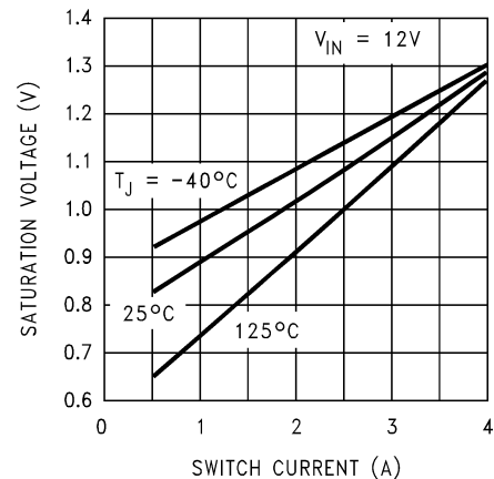
图 7-4. Switch Saturation Voltage
