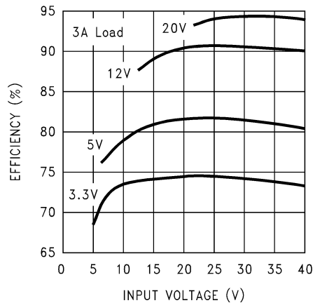
图 7-3. Efficiency
