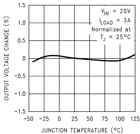
图 7-1. Normalized Output Voltage
