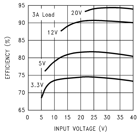
图 7-3. Efficiency
