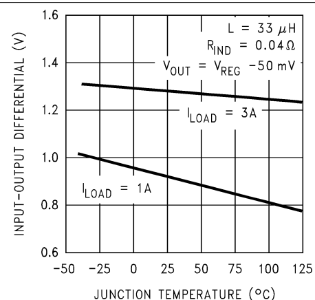
图 7-6. Dropout Voltage
