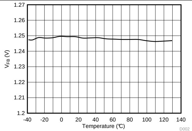
图 2. V_{FB} vs Temperature
