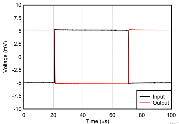
图 6-28. Overload Recovery
