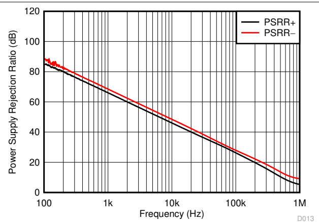
图 6-7. PSRR vs Frequency
