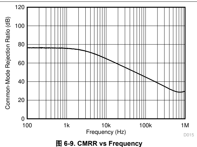
图 6-9. CMRR vs Frequency
