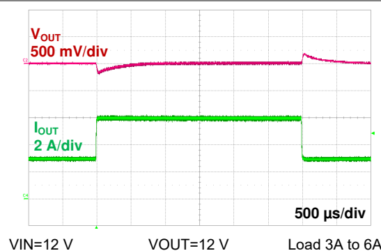
图 6-16. Load Step (Buck-Boost)
