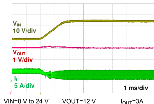
图 6-18. Line Transient
