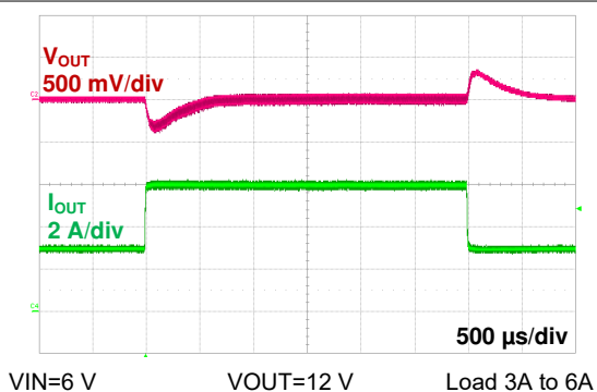
图 6-15. Load Step (Boost)
