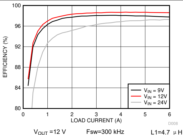
图 6-2. Efficiency vs Load
